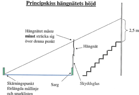
Principskiss hängnätets höjd
